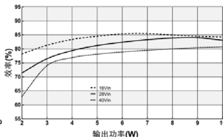
6: WK392815D-10 效率曲线
