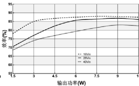
6: WK392815D-10 效率曲线
