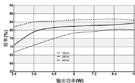
4: WK392805D-10 效率曲线
