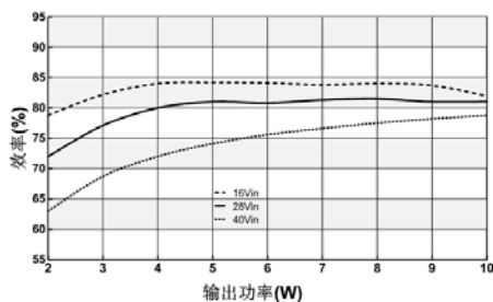
3: WK392815S-10 效率曲线
