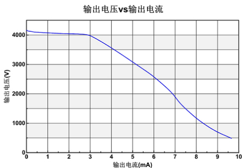
图 2 负载特性
