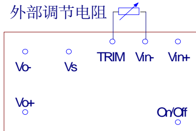
图 4 输出电压调节方式
