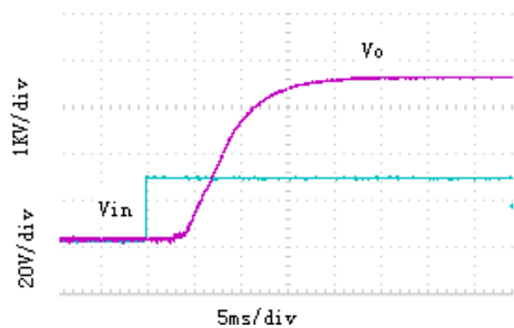
图 1 启动波形
