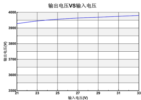
图 3 电压特性
